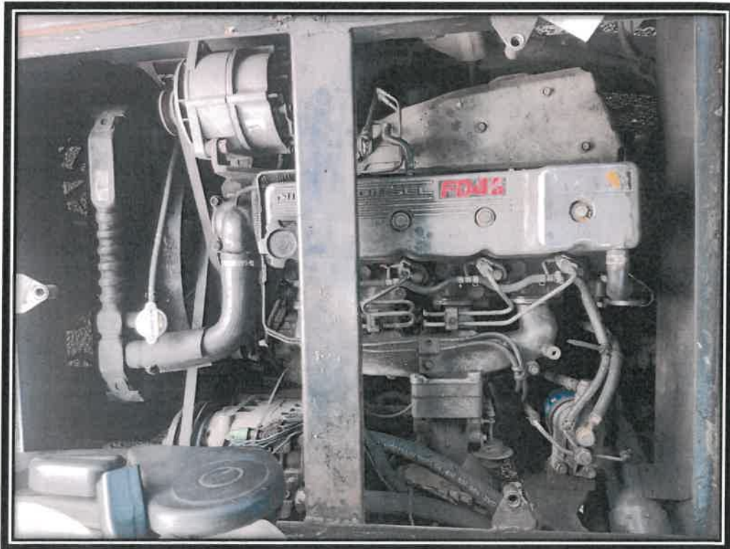
GAMBAR WRW 3475: BAHAGIAN ENJIN
